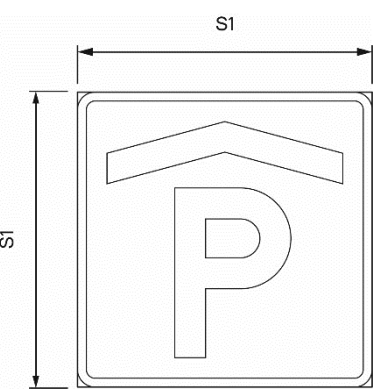
Storlek och mått i meter för märke F28
