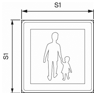
Storlek och mått i meter för märke E7 och E8
