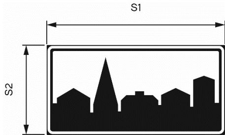
Storlek och mått i meter för märke E5 och E6
